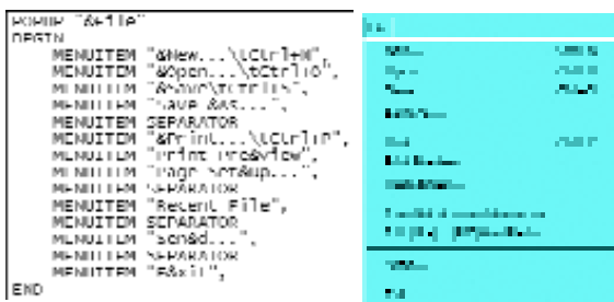
Abb.2: Menü im Quellcode (links) und in der kompilierten Programmdatei (rechts)
